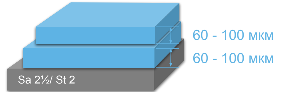
2-слойная система Толщина покрытия: 120-200 мкм
